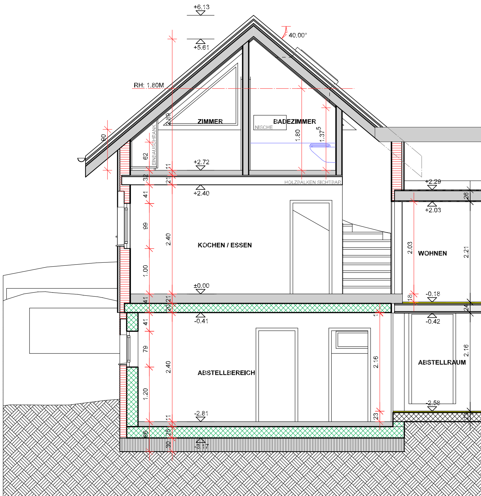
SCHNITT A-A
