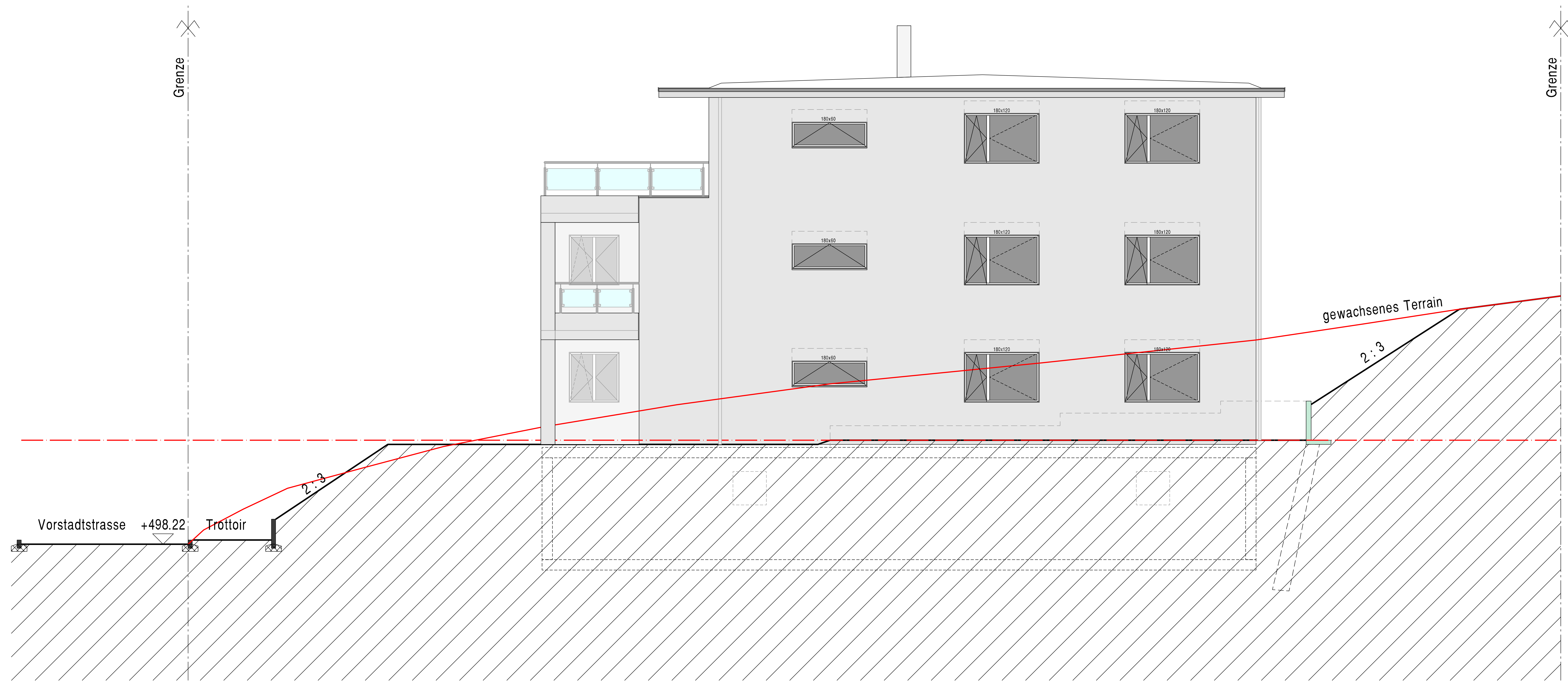
Ostansicht 1:100
