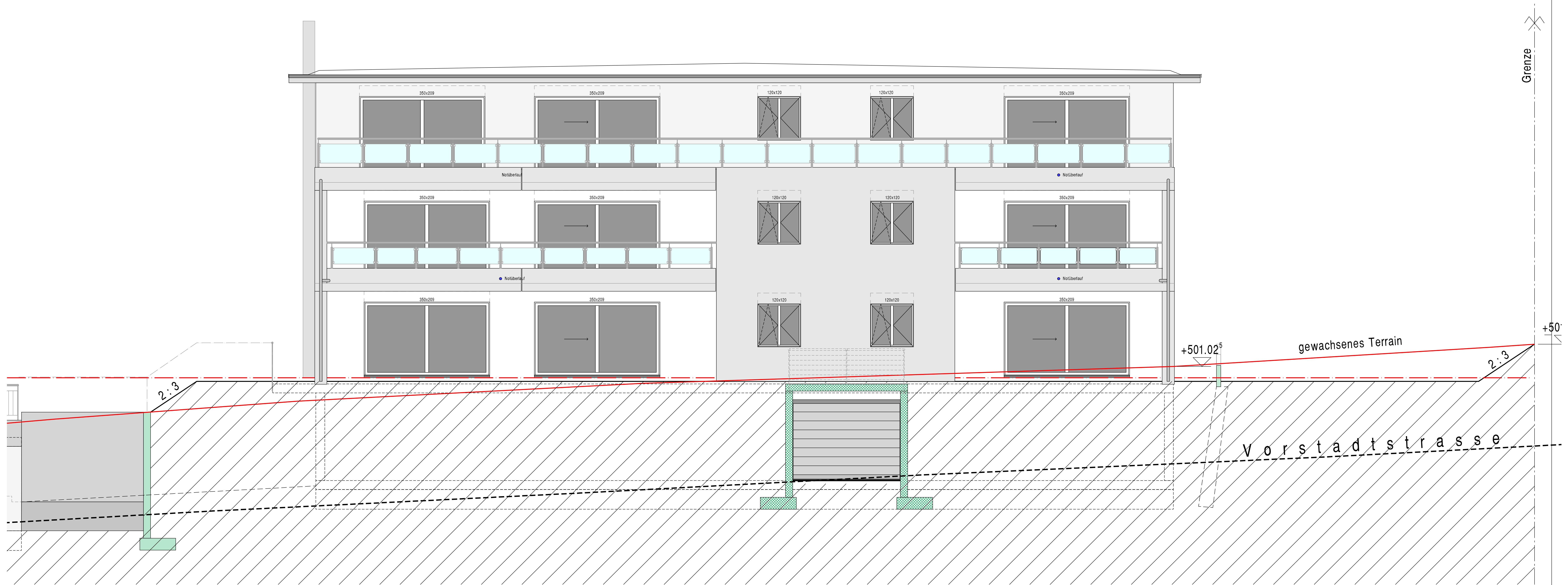
Südansicht 1:100
