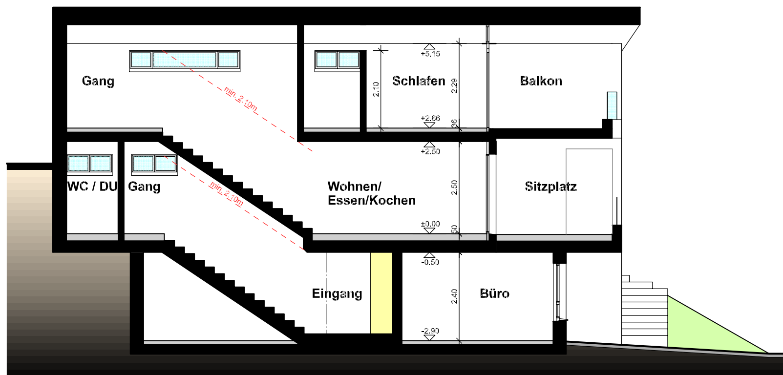
SCHNITT A-A
