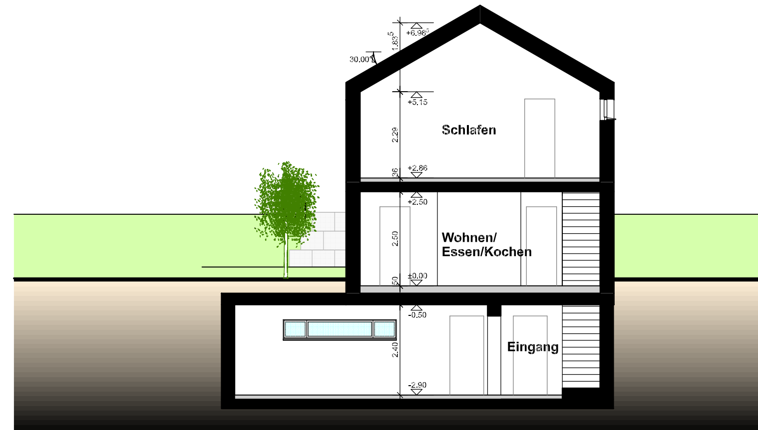
SCHNITT B-B
