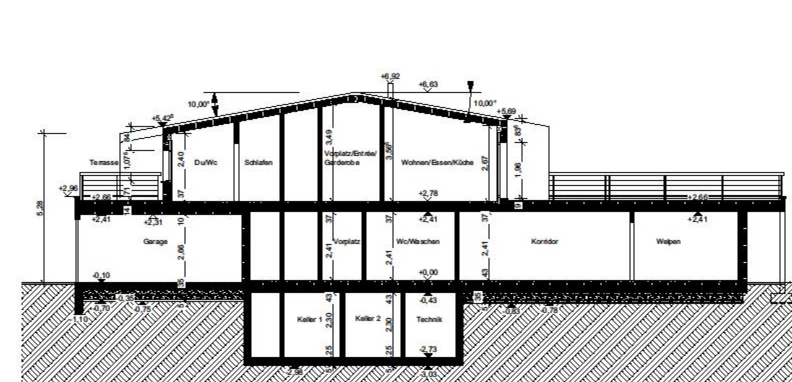
Schnitt Wohnhaus A-A
